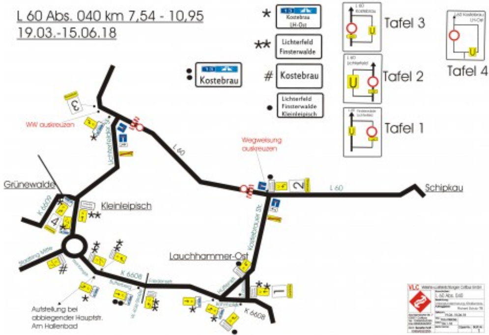
Umleitungsplanung für die L 60-Baustelle
