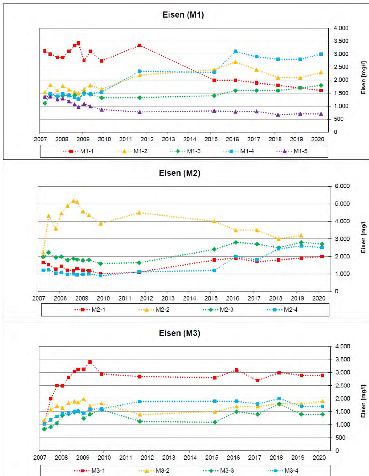
Abbildung 4: Konzentrationsentwicklung für Eisen gelöst (M1 bis M3)
