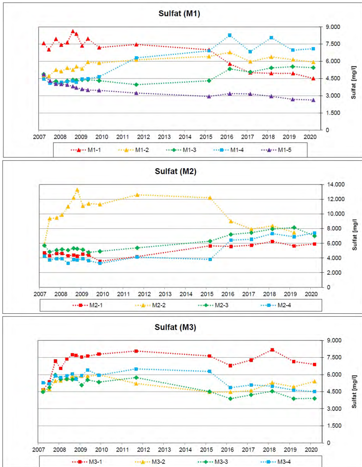
Abbildung 5: Konzentrationsentwicklung für Sulfat (M1 bis M3)
