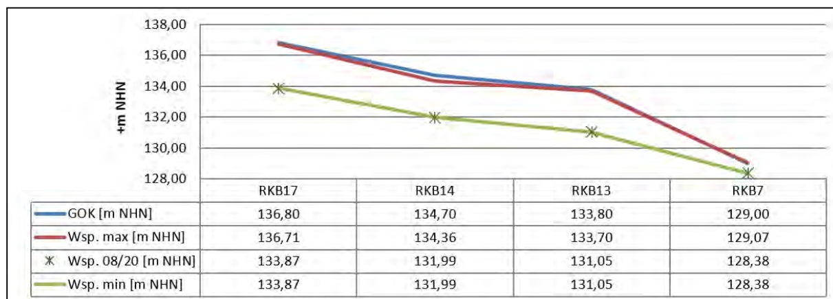
Abbildung 7: Wasserstände (Ist, Min und Max) im Profil I (Zeitraum 2007 bis 2020)
