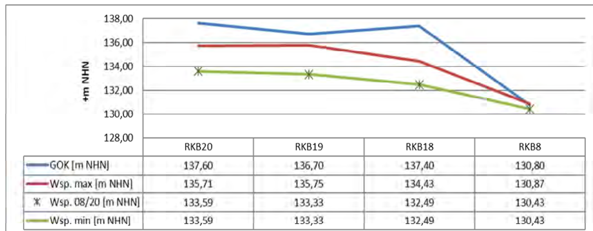
Abbildung 9: Wasserstände (Ist, Min und Max) im Profil III (Zeitraum 2007 bis 2020)
