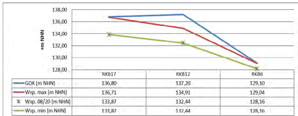
Abbildung 8: Wasserstände (Ist, Min und Max) im Profil II (Zeitraum 2007 bis 2020)
