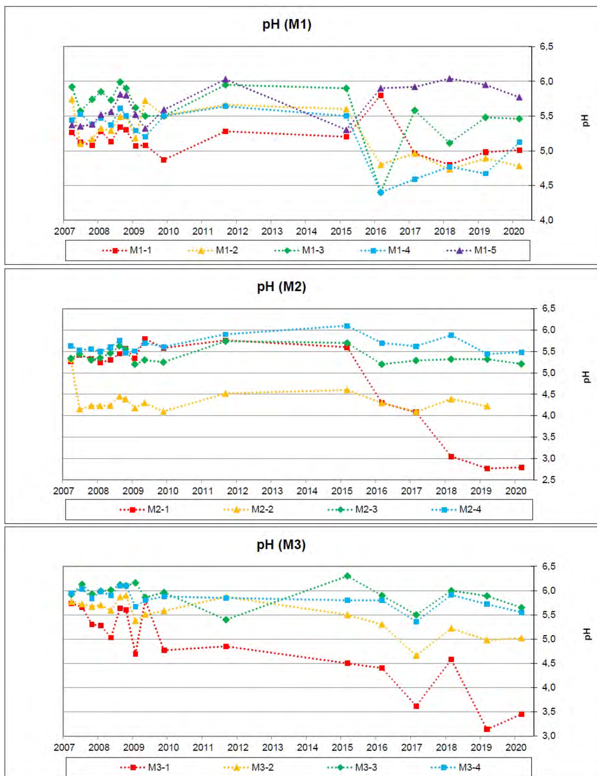
Abbildung 3: Konzentrationsentwicklung für pH-Wert (M1 bis M3)
