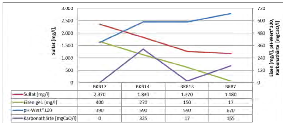
Abbildung 10: Konzentrationsverteilung im Profil I für pH, Eisen gelöst , Sulfat und Karbonathärte (Messwerte RKB14 aus 2017)
