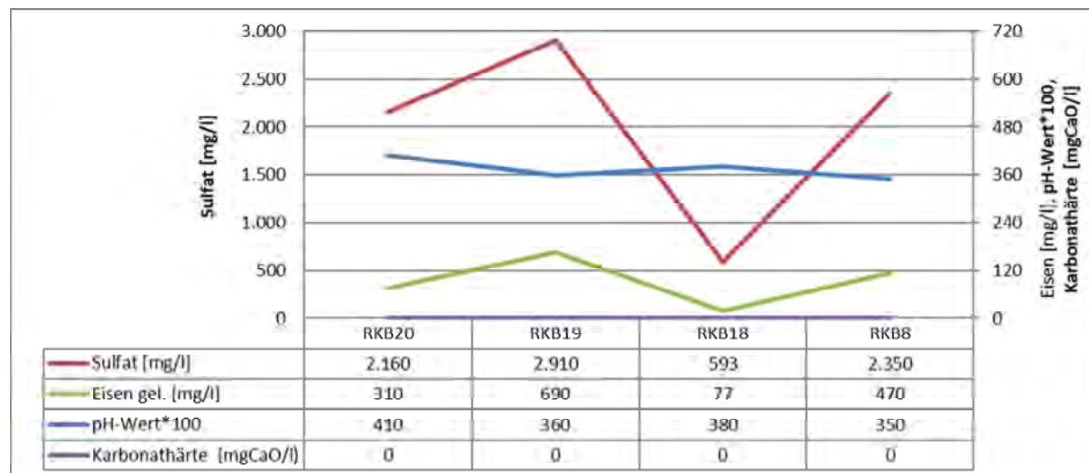
Abbildung 12: Konzentrationsverteilung im Profil III für pH, Eisen gelöst , Sulfat und Karbonathärte (Messwerte RKB18 und RKB20 aus 2017)
