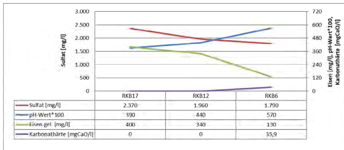
Abbildung 11: Konzentrationsverteilung im Profil II für pH, Eisen gelöst , Sulfat und Karbonathärte (Messwerte RKB12 aus 2018)
